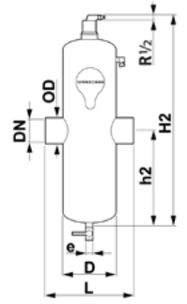
Kaynaklı Bağlantı
